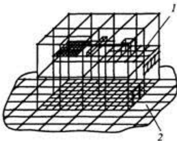
Рис. 4.7. Сетчатое заземляющее устройство здания: 1 - сеть соединений; 2 - заземлитель
