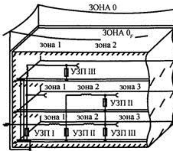
Рис. 4.9. Пример установки УЗП в здании
