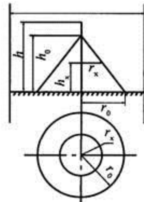
Рис. 3.1. Зона защиты одиночного стержневого молниеотвода
