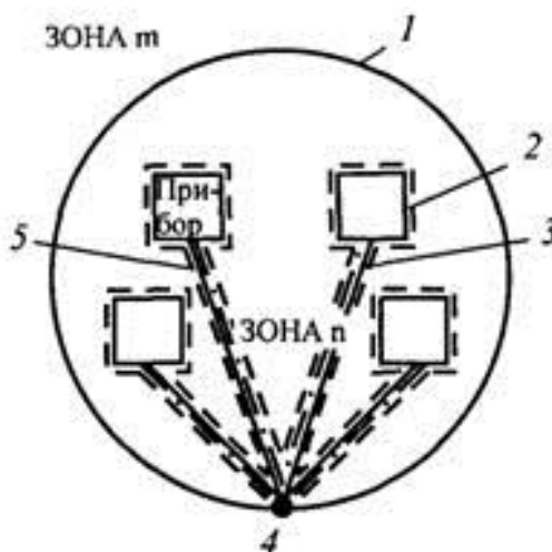
Рис. 4.4. Схема соединения проводов электропитания и связи при звездообразной системе уравнивания потенциалов: 1 - экран защитной зоны; 2 - электрическая изоляция; 3 - провод системы уравнивания потенциалов; 4 - центральная точка системы уравнивания потенциалов; 5 - провода связи, электропитания
