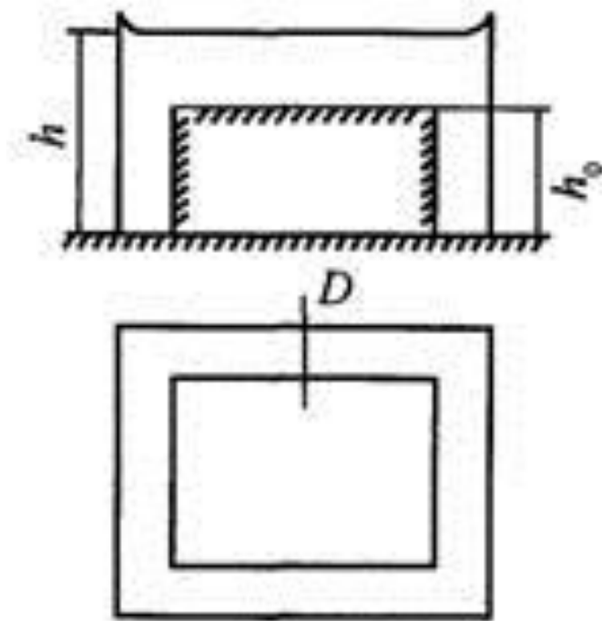
Рис. 3.5. Зона защиты замкнутого тросового молниеотвода
